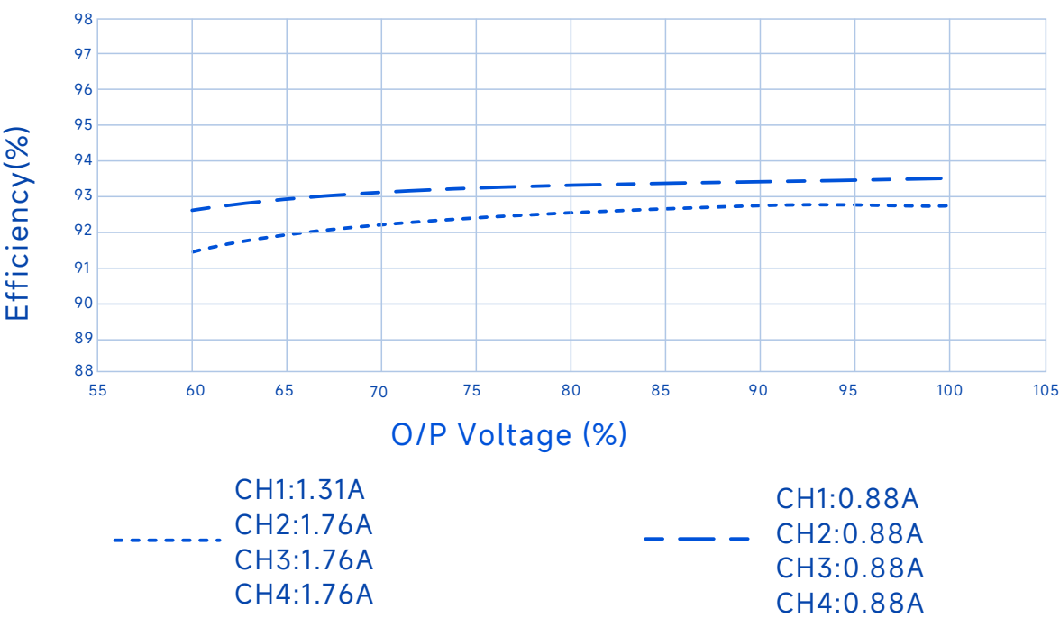
效率Vs.输出电压(Vin=400Vac)
