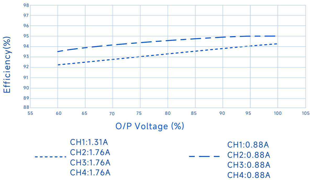
效率Vs.输出电压(Vin=400Vac)
