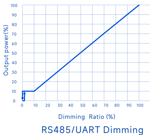
输出功率Vs.调光信号
