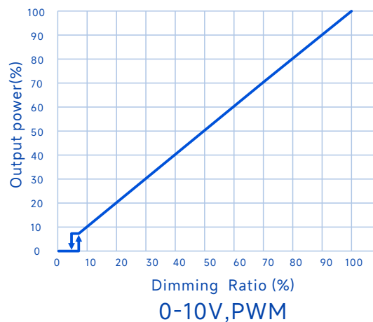
输出功率Vs.调光信号
